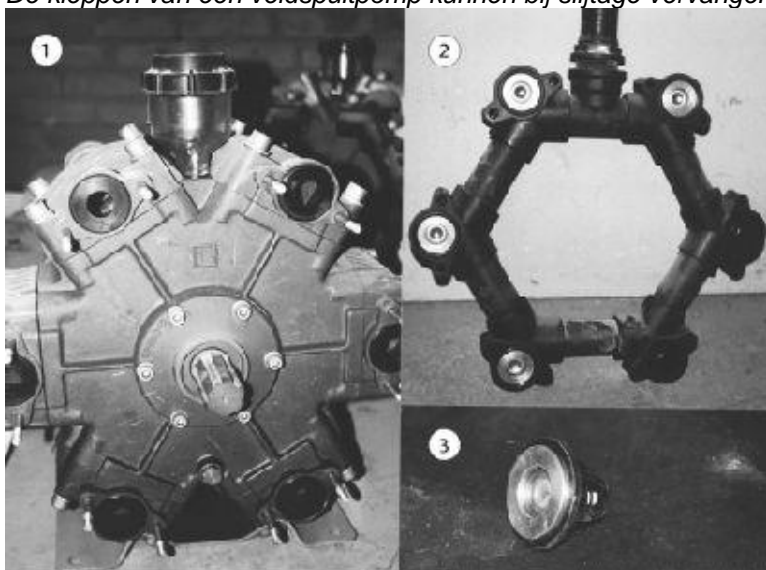
1: pomp 2: ring met kleppen 3: losse klep
